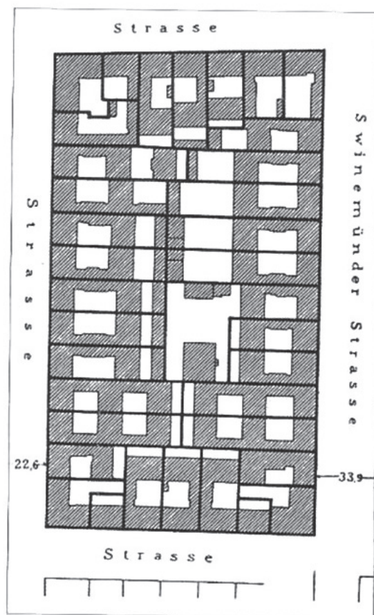
Figure 16: Tenement block with inner courtyards. Average floor plate 56m x 20m (Source: R. Eberstadt (1910). Handbuch des Wohnungswesens & der Wohnungsfrage, p.66)
