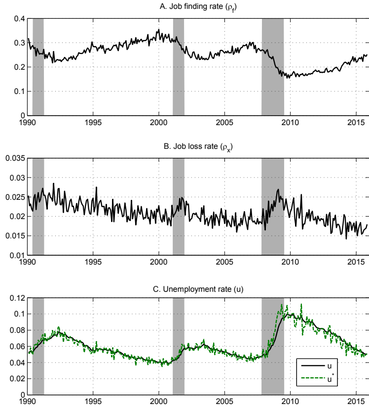
Figure 2: Raw data.
